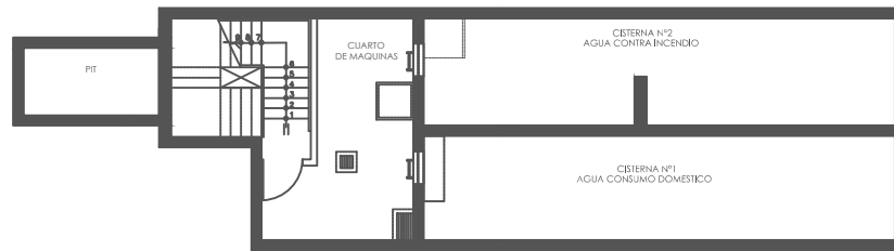
PISO SOTANO 2 1/200
